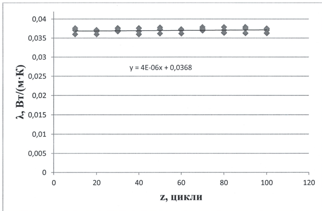
Рисунок 3 – Залежність теплопровідності від циклічних впливів
